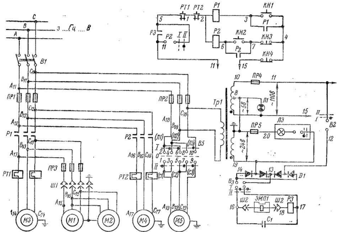
Рис. 14. Схема электрическая принципиальная
